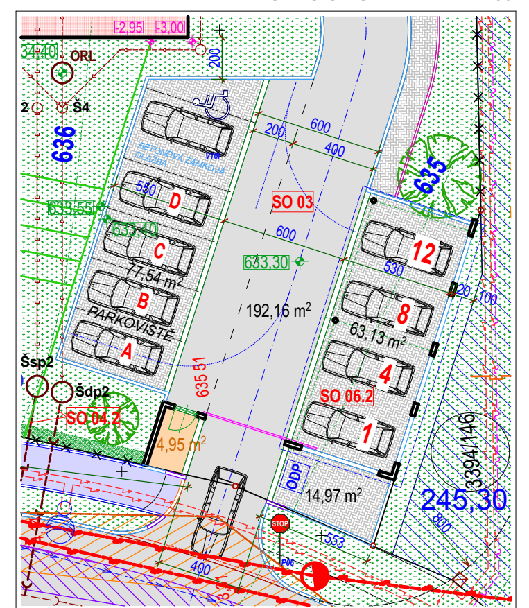
SCHÉMA VENKOVNÍCH KRYTÝCH PARKOVACÍCH STÁNÍ M 1:250
